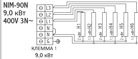
Рис. 5 Fig. 5 Схема электроподключения Electrical Diagram
